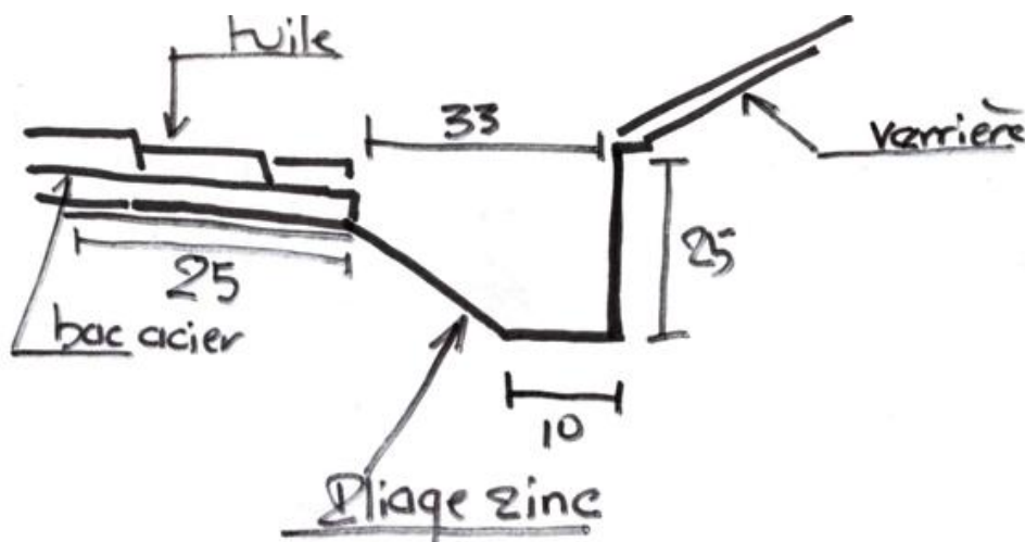
Détail du chéneau B
