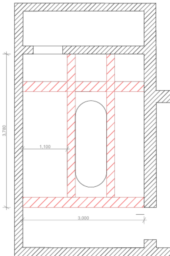
PLAN VERRIERE EXISTANTE
